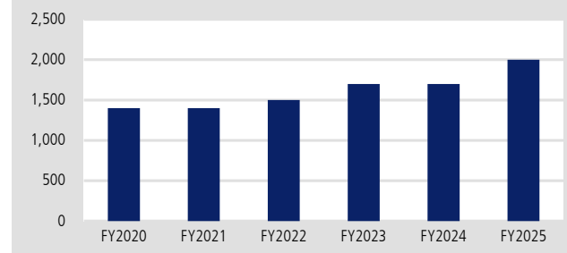
圖 19 : Walmart - 捐款額
