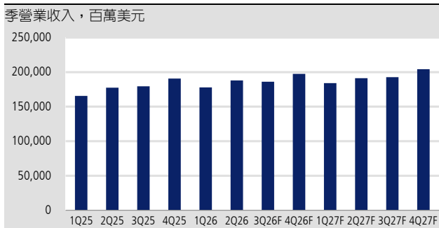
圖 8：季營業收入
