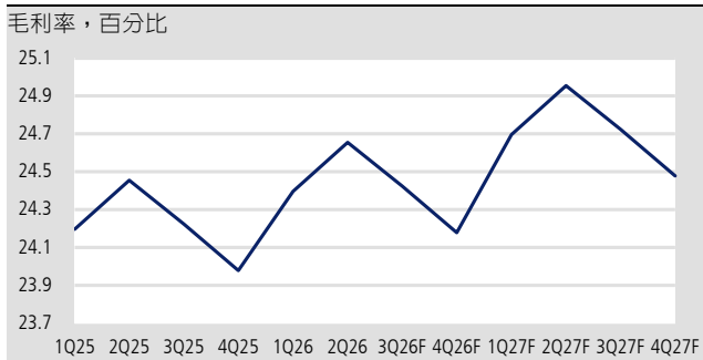
圖 10：毛利率
