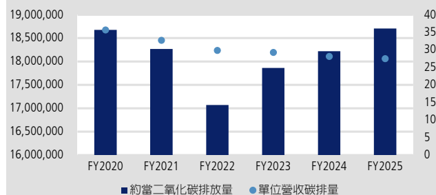
圖 18 : Walmart - 碳排量
